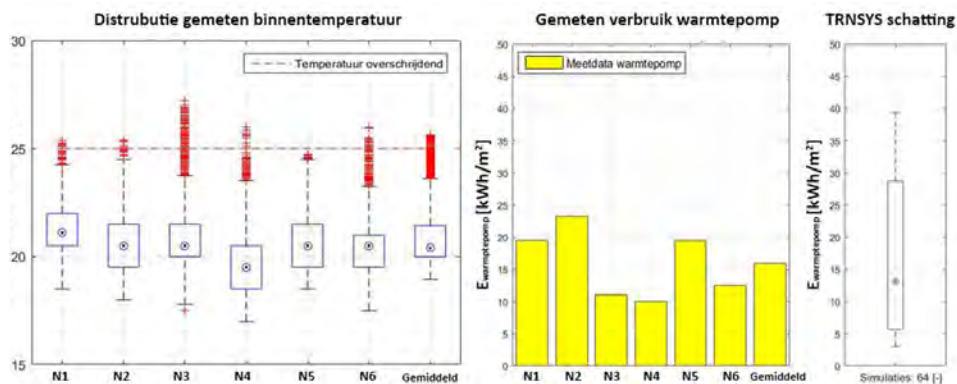
-Figuur 3- Verschil in het binnenklimaat (links) en het gebouwgebonden elektriciteitsverbruik van de warmtepomp zowel gemeten (midden) als gemodelleerd in TRNSYS 17 (rechts) voor zes rijwoningen in Holten gedurende de tijdsperiode van januari tot en met juli 2015
