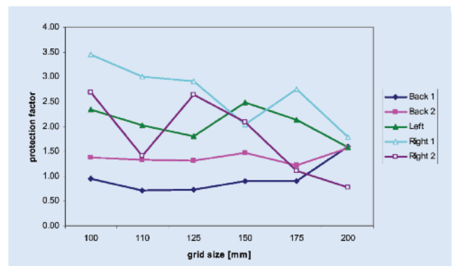
Protectiefactor op de instrumentafels als functie van de celgrootte.
