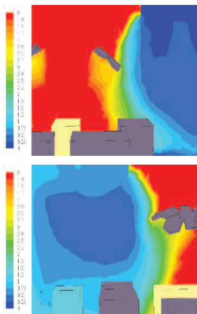
Voorbeeld van een berekende protectiefactor voor een verticale doorsnede in de operatiekamer (links: instrumenttafel aan de linkerzijde van de operatietafel; rechts: instrumenttafel aan het voeteneinde van de operatietafel).
