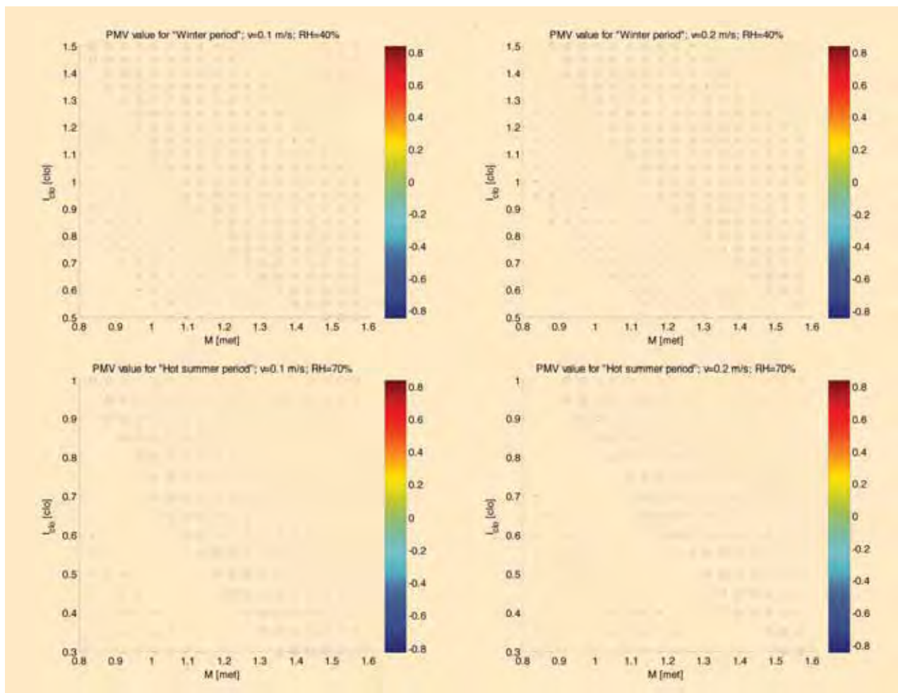
Oplossing voor het zoekgebied voor het metabolisme ( M ) en de kledingweerstand ( I_{clo} ) voor de volgens het ATC-model toegestane operationele temperatuurrange bij 80 % acceptatie voor de bij de grafieken aangegeven condities ('x' relateert aan de bovengrens voor de operationele temperatuur en 'o' aan de ondergrens).
