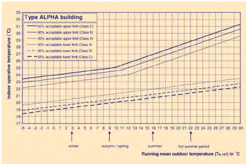
Maximaal toelaatbare range van de operationele binnentemperatuur voor een specifiek acceptatieniveau, als functie van een lopend gemiddelde van de buitentemperatuur ( T_{e,ref} ), voor een type Alpha-gebouw [9].
